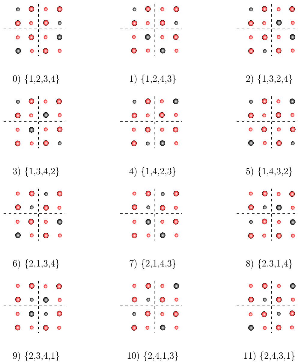
Рис. 1: Атомы у ядра исходной конфигурации в плане
